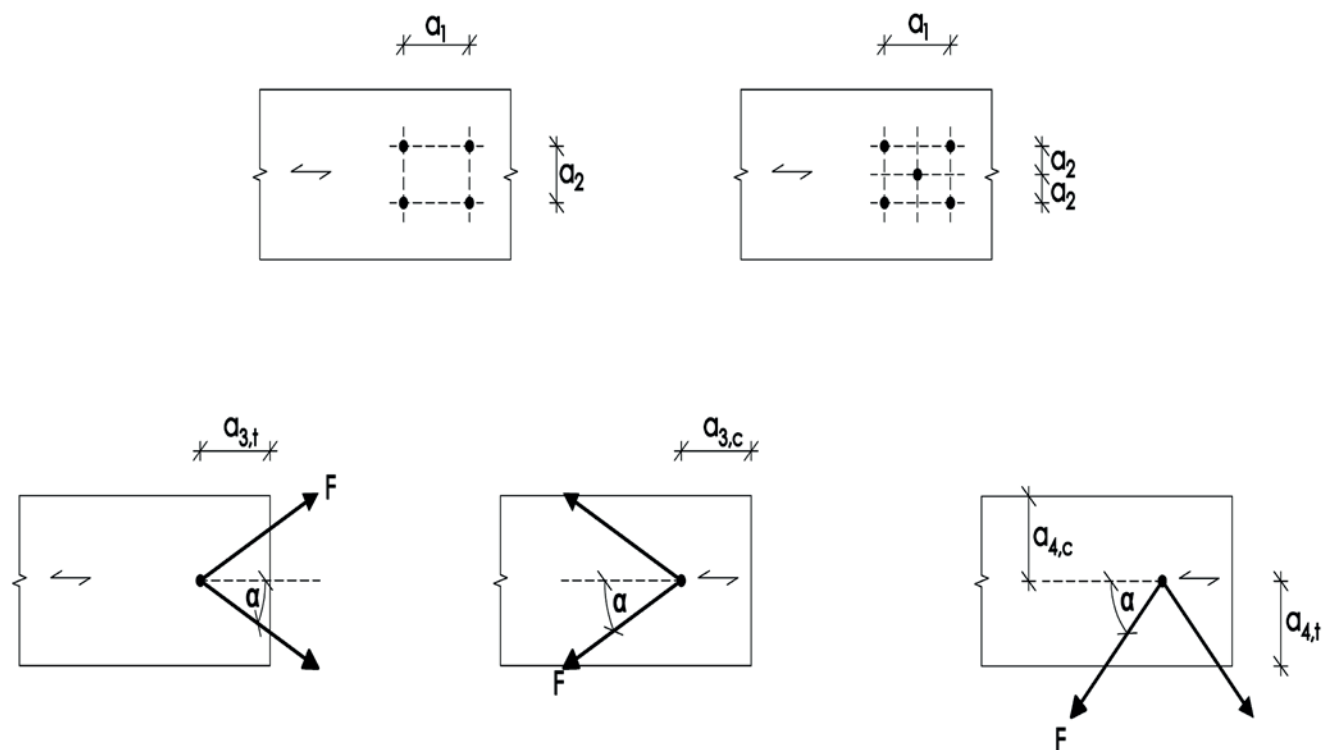
Abbildung E.1: Definition der Achs-, End- und Randabstände in der Seitenfläche
